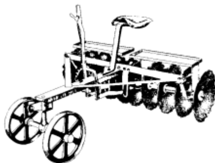
Figura 5. Grade de discos para tração animal. Fonte: REIS (1983).
